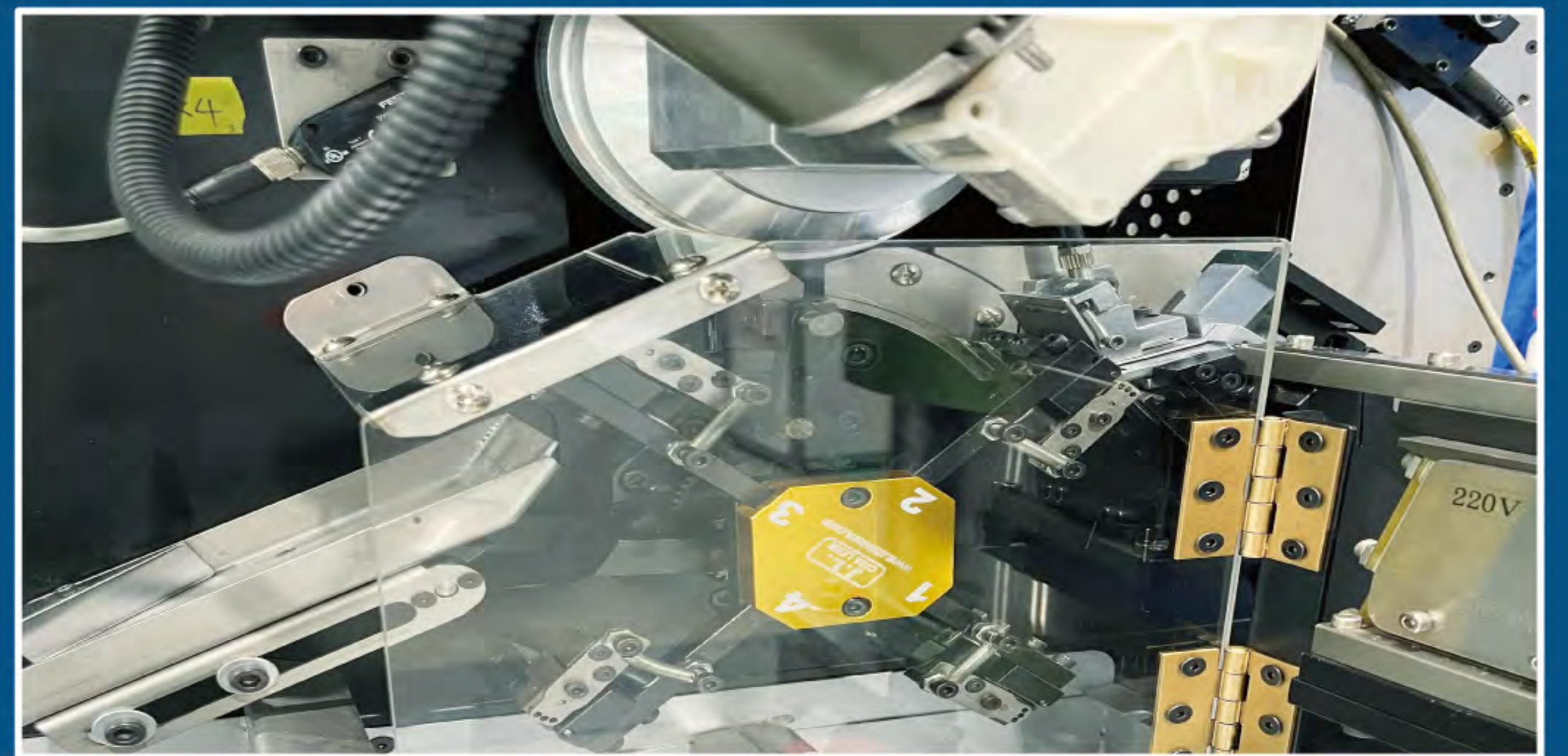
◎ 摩天輪式進出料設計 Ferris wheel load and unload design
